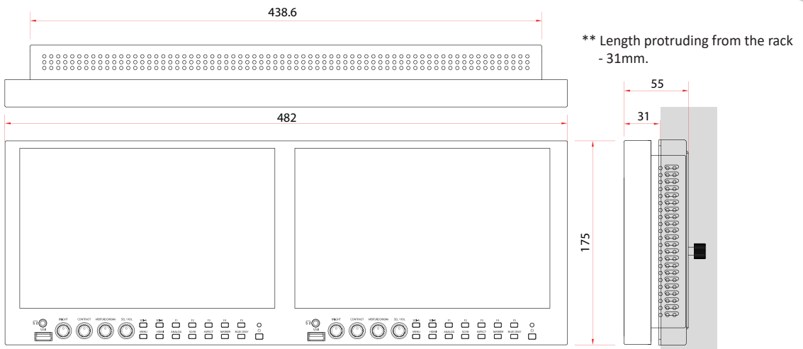
PRM-102F Dimensions(mm)
