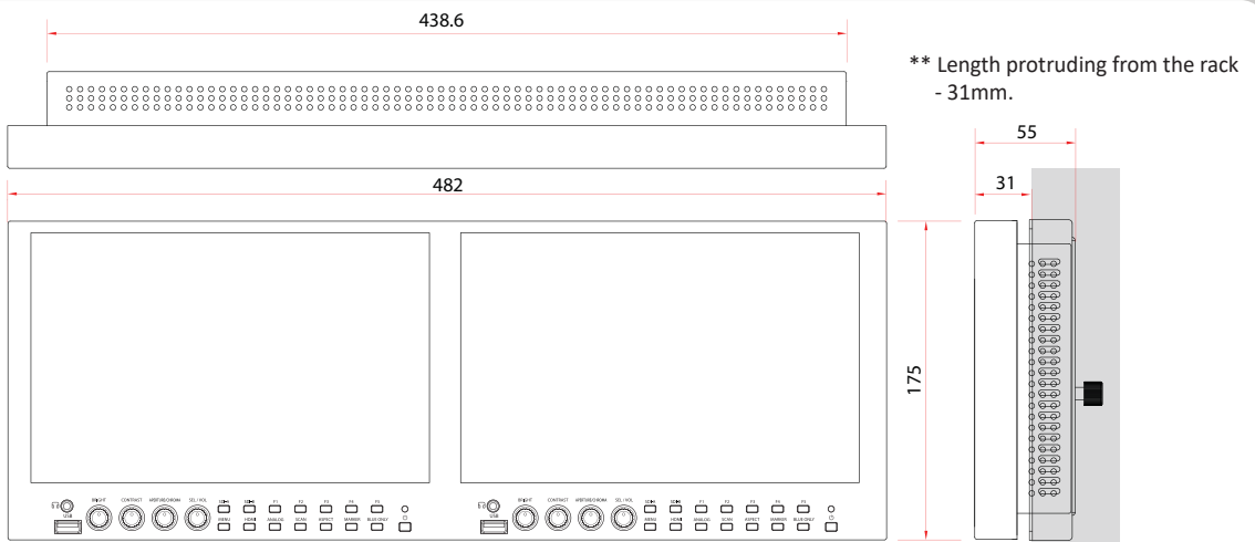
PRM-102F Dimensions(mm)
