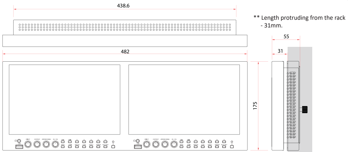
PRM-102F Dimensions(mm)
