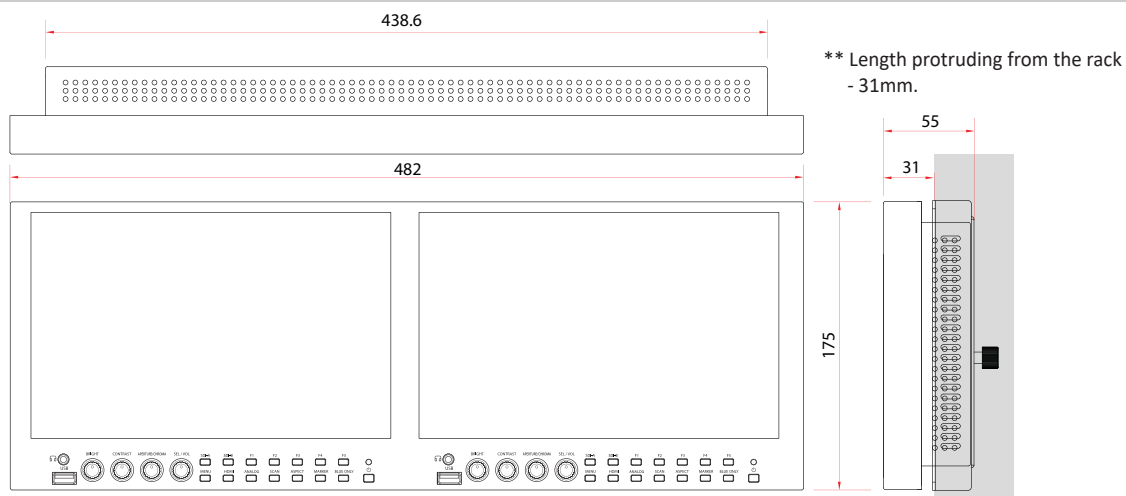
PRM-102F Dimensions(mm)
